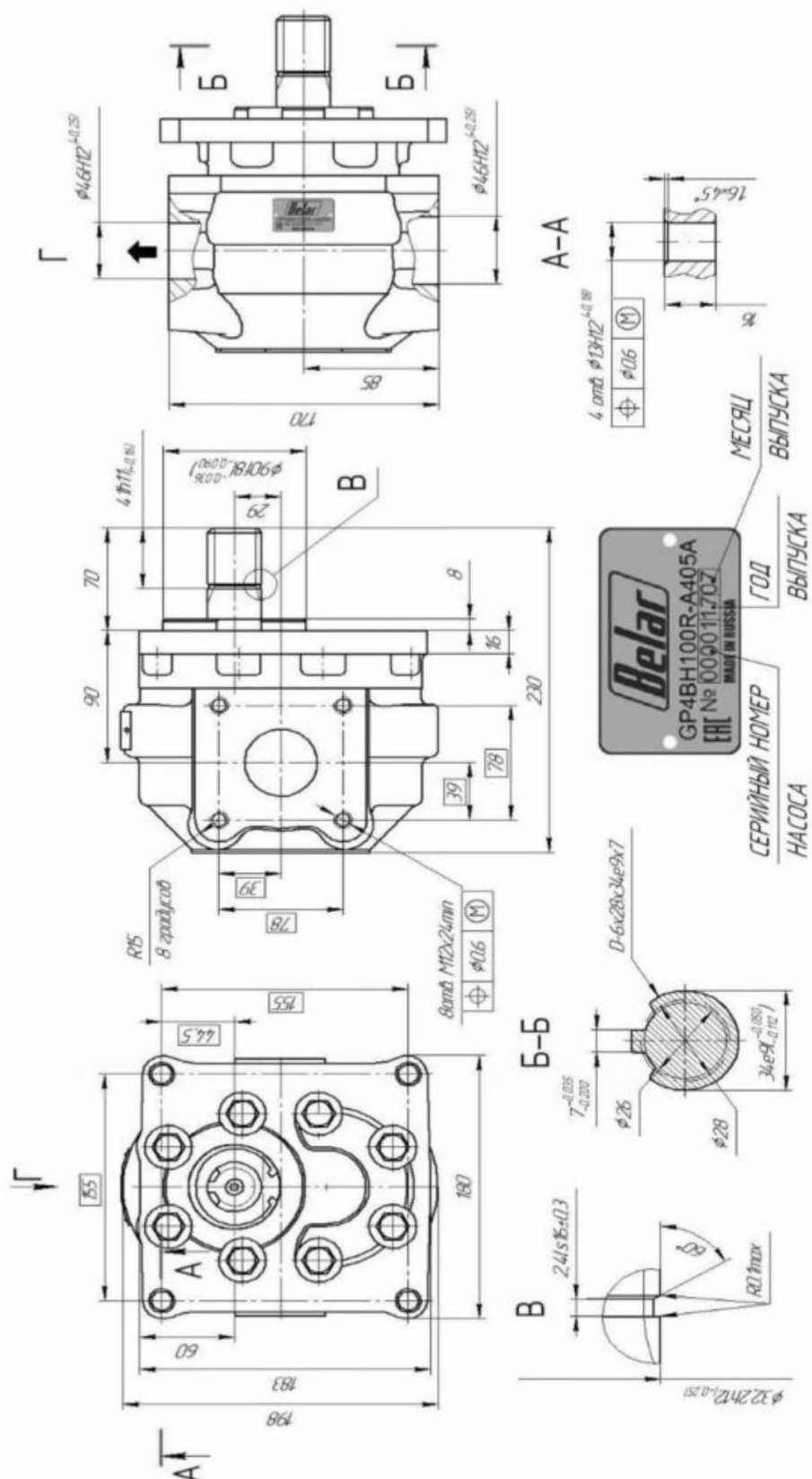
Рис.3 Габаритные и присоединительные размеры шестеренного насоса GP4BH100R
