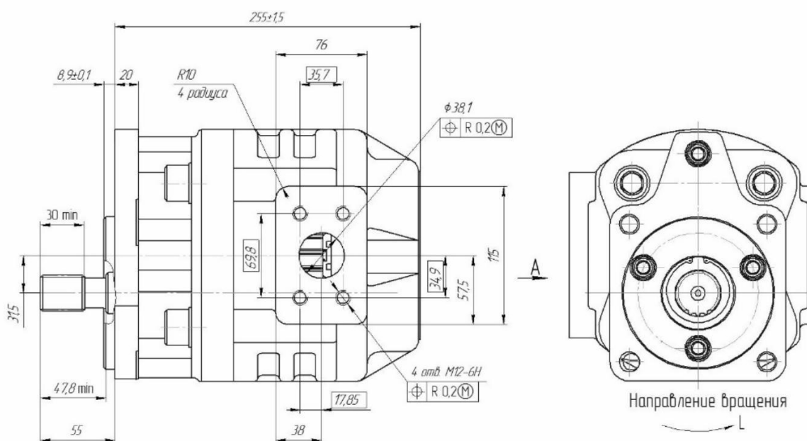
Рисунок 4. Габаритные и присоединительные размеры GP4BF150L-B736W 21. (остальное см. рисунок 3)
